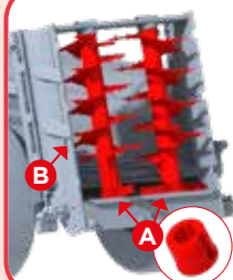
Wałki \varnothing 820 lub 900 mm zależnie od modelu, zwoje 10 mm.
