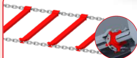
Listwy rurowe przyspawane do łańcuchów ogniowych 14 (zapobieganie osadzaniu się materiału) + zębaki spawane.
